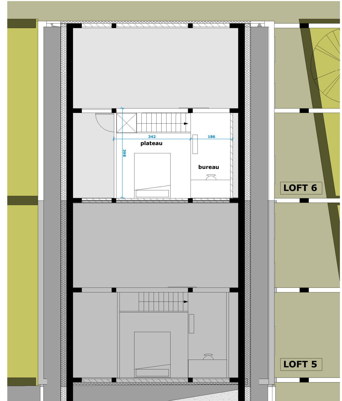
Verdieping
