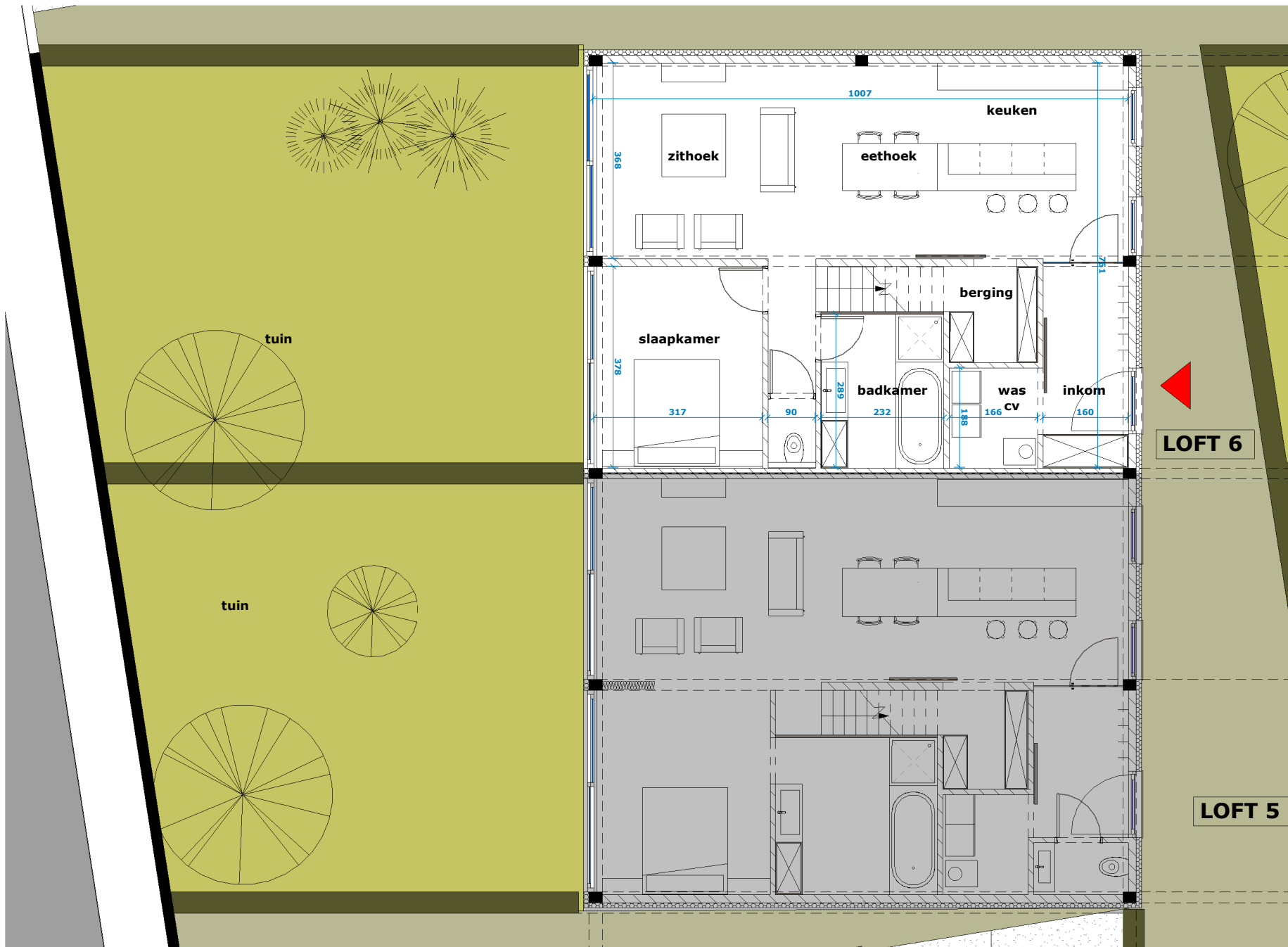
Gelijkvloers
